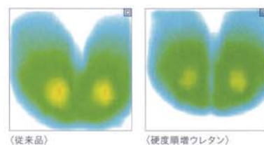
■耐圧分散計測図
