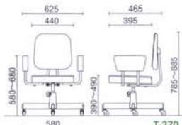
T-270 レザー ¥28,200* 質量:12.2kg 仕様:背ロッキング・手動上下調節 塗装脚
