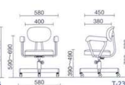
T-230 レザー ¥20,600* 質量:8.4kg 仕様:背ロッキング・手動上下調節 塗装脚
