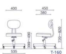
T-160 レザー ¥14,000* 質量:6.8kg 2本入 仕様:背ロッキング・手動上下調節 塗装脚
