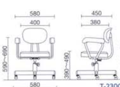
T-230CG レザー ¥23,500* 質量:8.4kg 仕様:背ロッキング・手動上下調節 クロームメッキ
